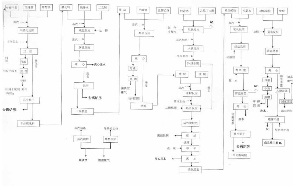
泛醇工艺流程图
